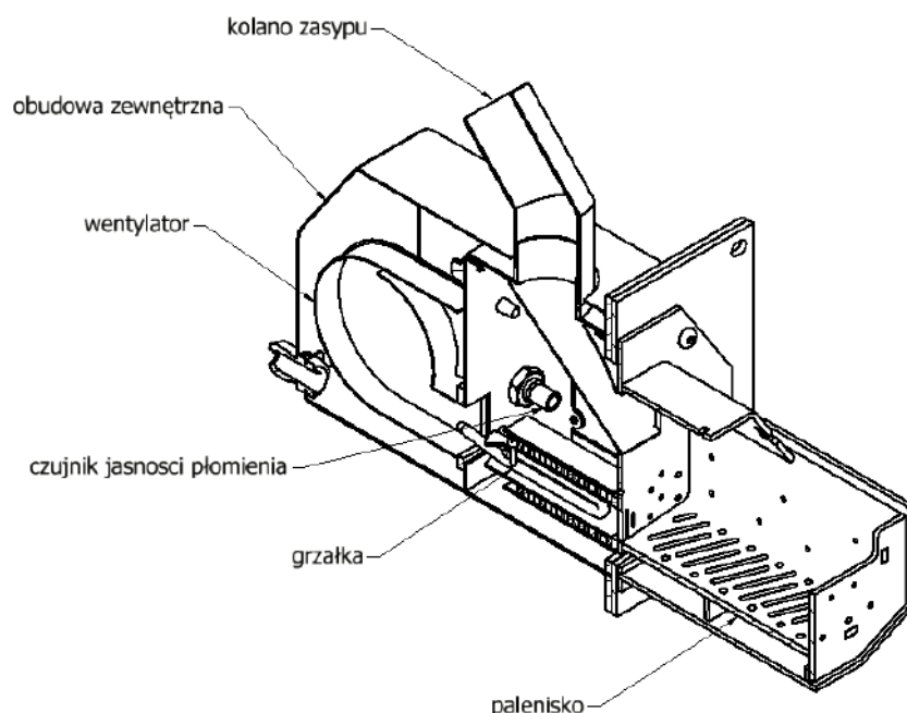
Rys.4 Budowa palnika
