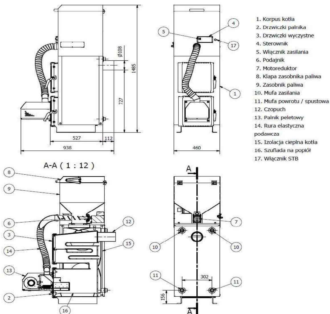
Rys. 1 Wymiary i opis kotła PELL DUO+ 10 kW opcja zbiornik u góry
