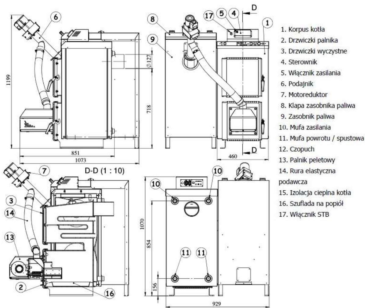
Rys. 2 Wymiary i opis kotła PELL DUO+ 10 kW opcja zbiornik z boku
