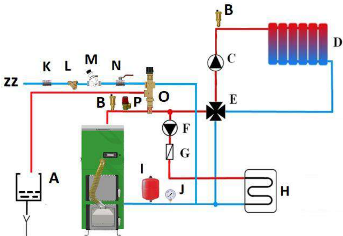
Rys. 10 Uproszczony schemat instalacji grzewczej systemu zamkniętego
