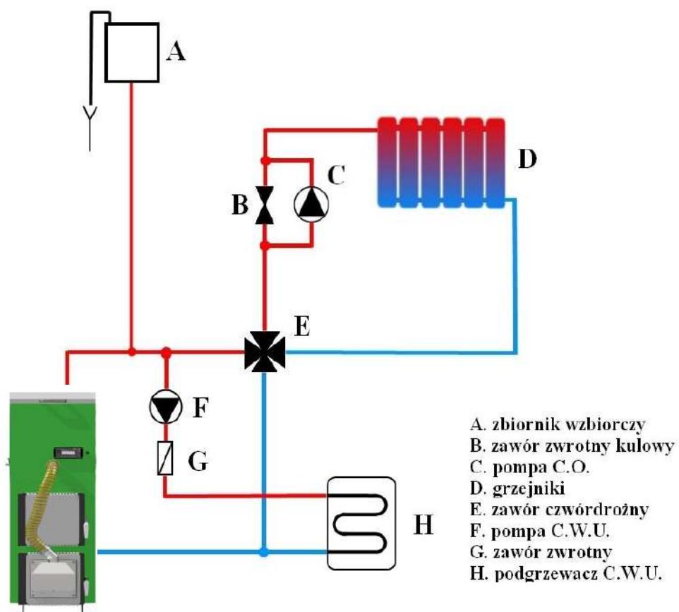
Rys. 9 Uproszczony schemat instalacji grzewczej systemu otwartego
