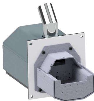
Rys. 3 Palnik duży moc 18-28kW
