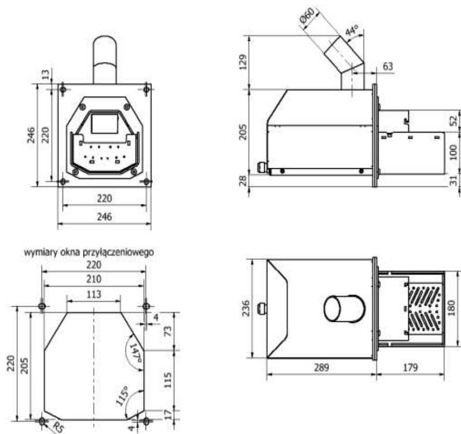
Rys. 5 Wymiary palnika
