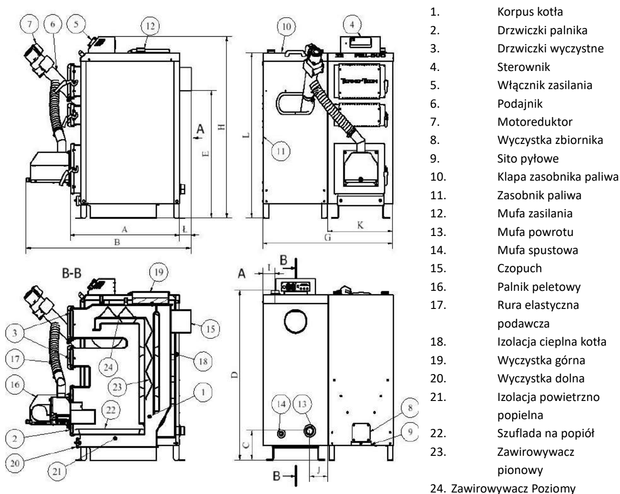
Rys. 1 Wymiary i opis kotła PELL-DUO+
