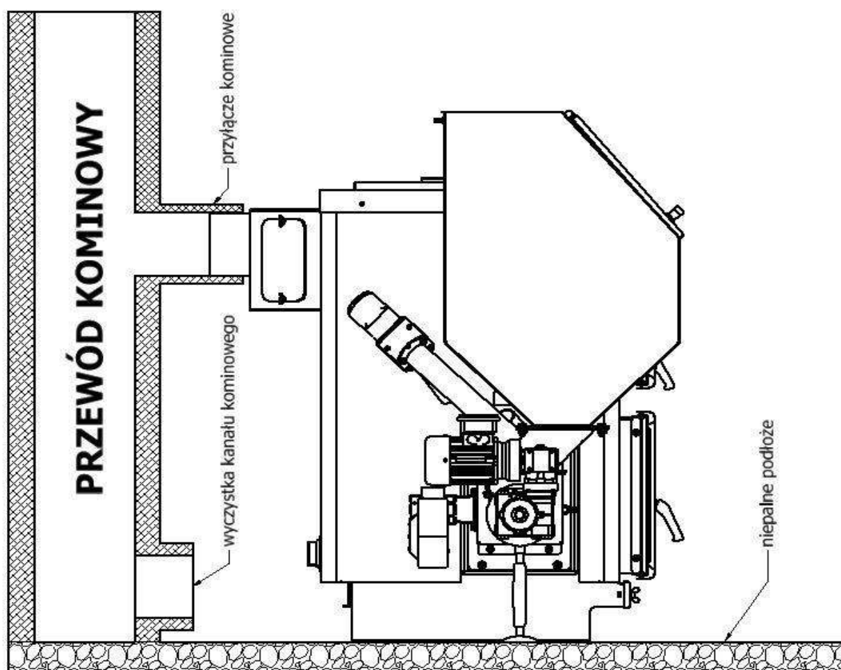
Rys. 3 Podłączenie kotła do komina
