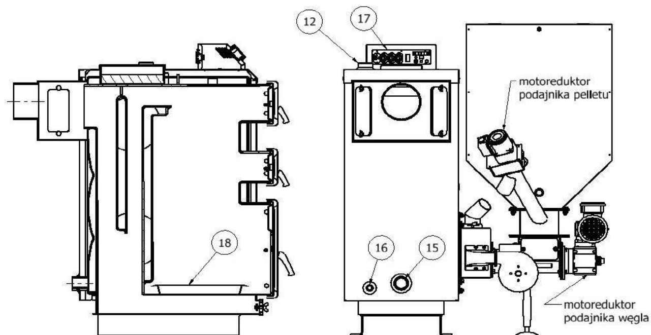
Rys. 1 Budowa kotła KRS EKO-PELL
