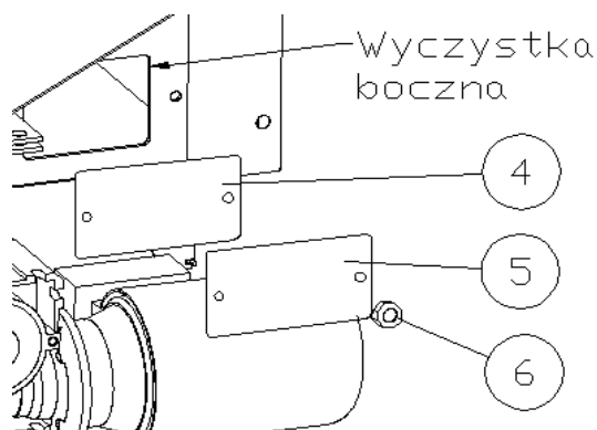
Rys. 9 Czyszczenie kotła przez wyczystkę boczną
