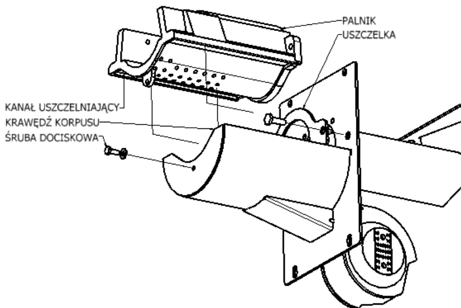
Rys. 10 Czyszczenie podajnika paliwa stałego
