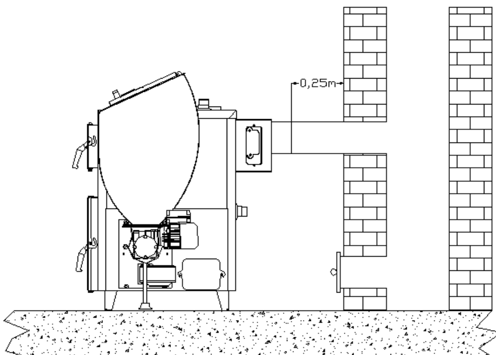
Rys. 3 Podłączenie kotła do komina
