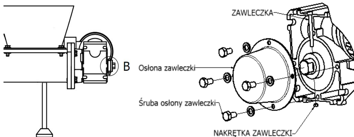
Rys. 6 Sposób montażu zawleczonej motoreduktora ze ślimakiem
