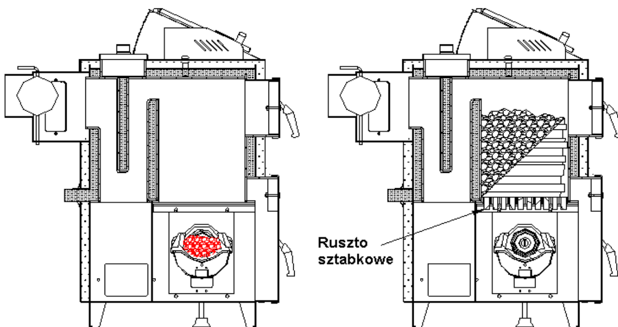
Rys. 7 Przekrój kotła i obiegi spalin przy spalaniu automatycznym (lewy) i ręcznym (prawy)
