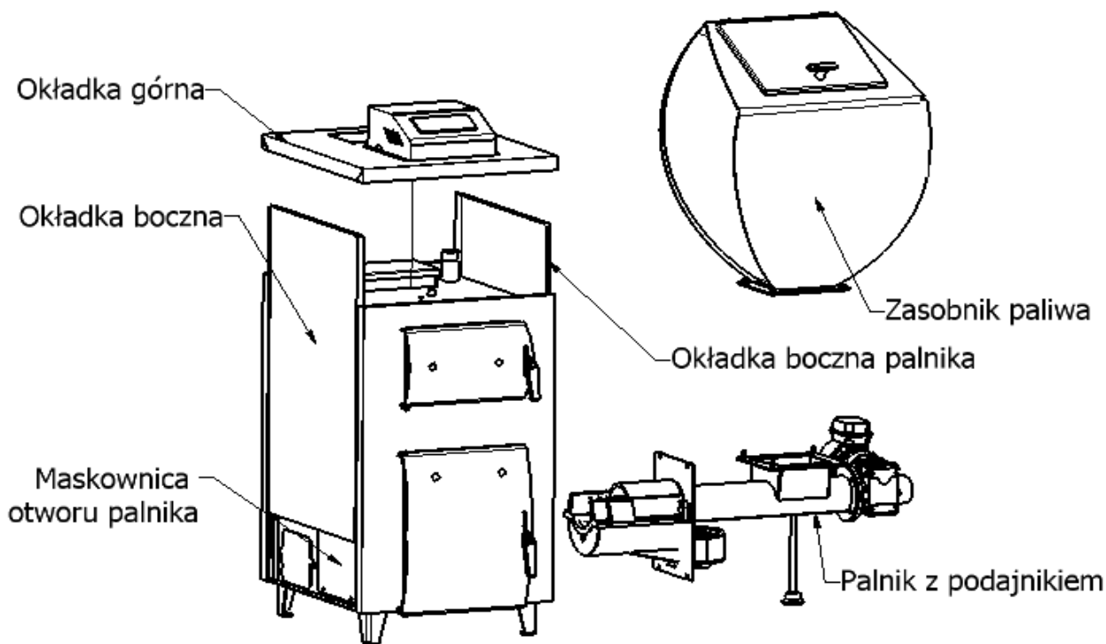
Rys. 11 Przekładanie podajnika na drugą stronę kotła
