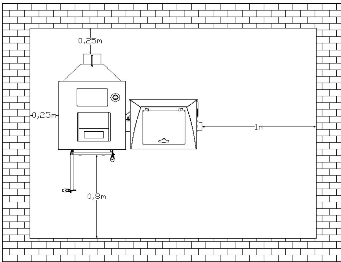
Rys. 2 Usytuowanie kotła w kotłowni
